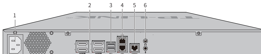
图1-3 TL-TUMS1500-MU后面板示意图
